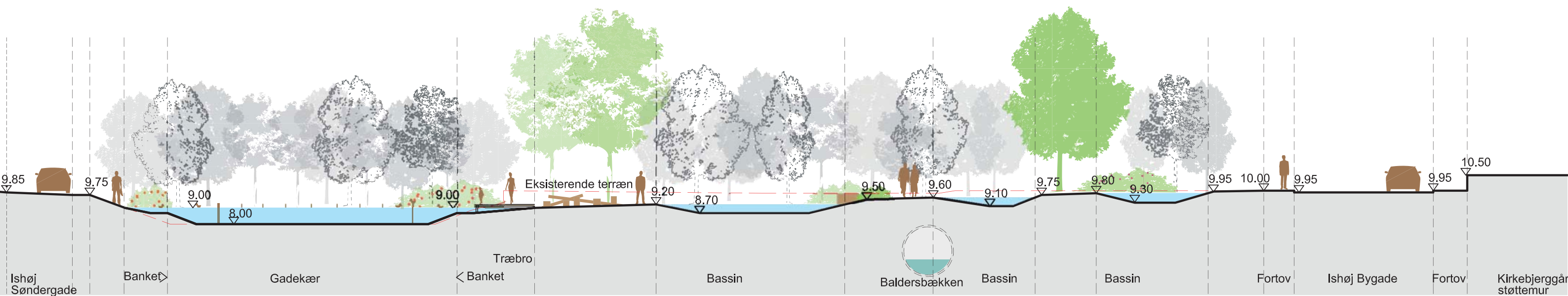
Principsnit Alternativ 1.
